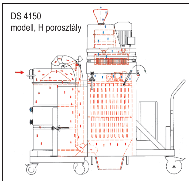
Elő leválasztó a különálló alvázon
